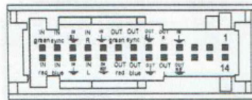
VW 26 pin plug
